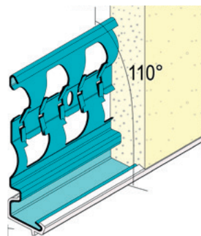
Abb. 4 Putzabschluss-/Sockelprofil.
